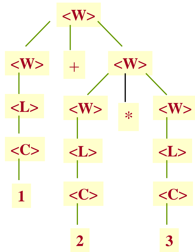
Poprawne drzewo rozbioru 1 + 2 * 3 = 7
