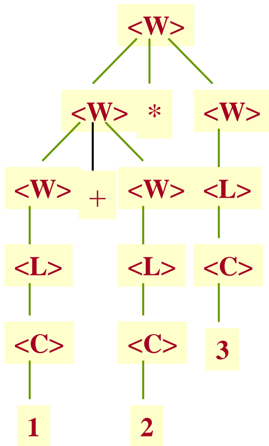
Niepoprawne drzewo rozbioru 1 + 2 * 3 = 9
