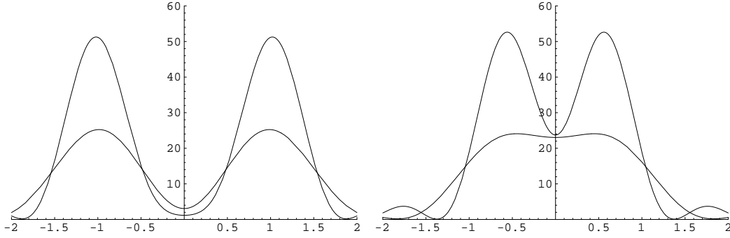
Rysunek 2: Wykres |a_m^{(1)}(t)|^2 jako funkcji \omega_{mn} dla dwu różnych czasów. Po lewej stronie duże \omega , po prawej mniejsze.
